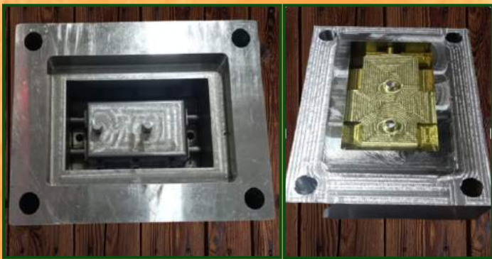
Compression die
