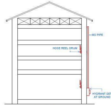
ELEVATION B
