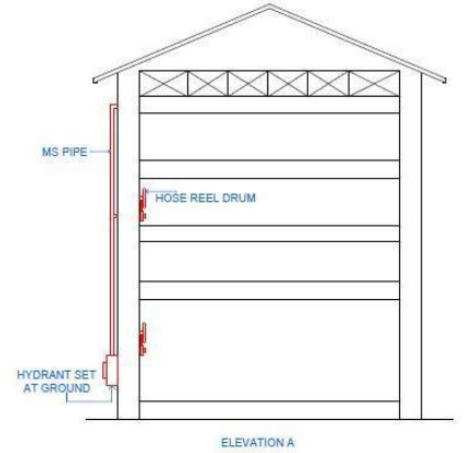
ELEVATION A
