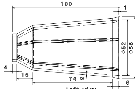
Left view Scale: 1:1
