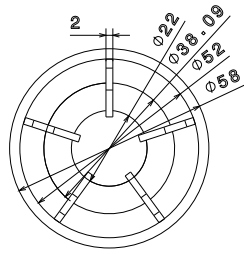
Top view Scale: 1:1
